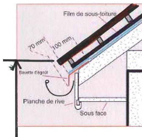
Hauteur à l'égoût ; ligne basse d'un pan de couverture
